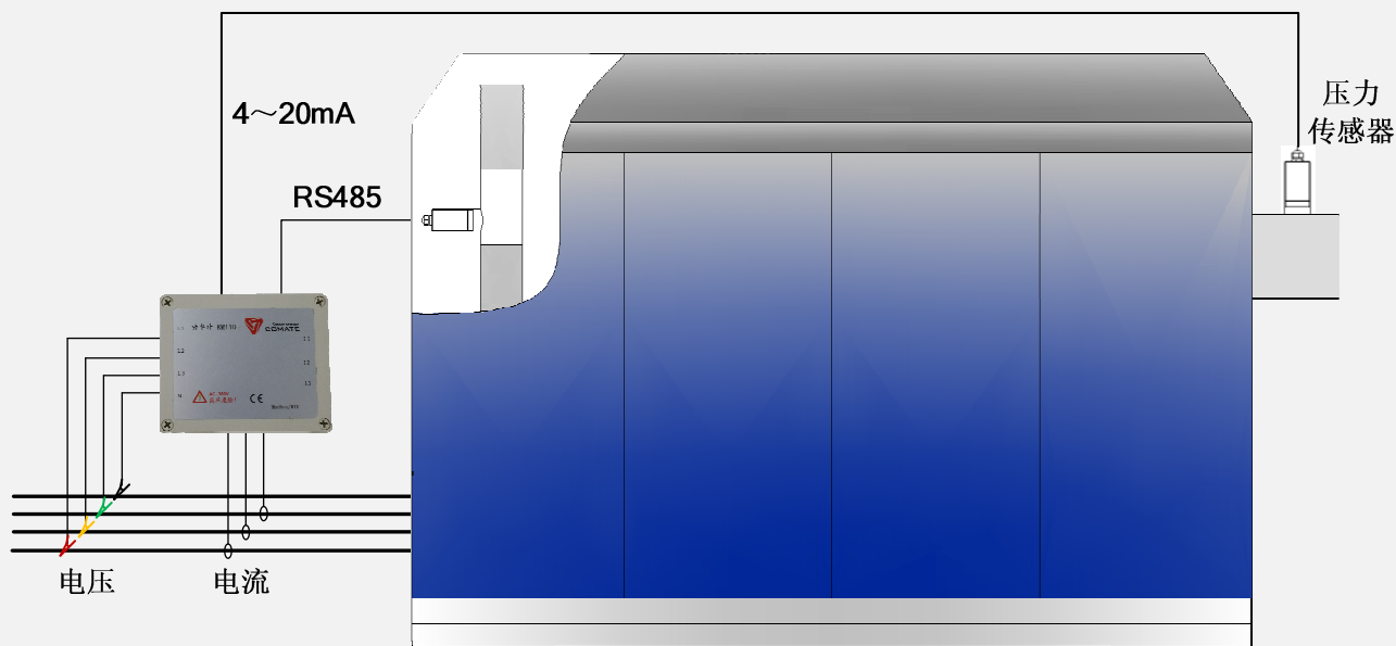
单台空压机接线图
